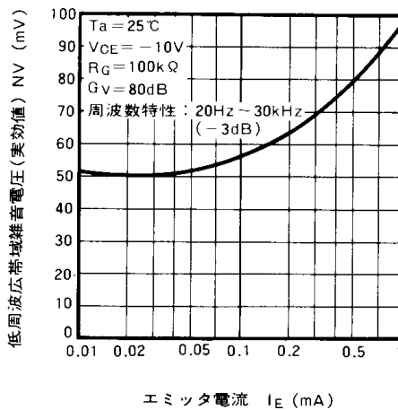
低周波広帯域雑音電圧(実効値)— エミッタ電流特性
