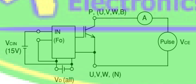
Fig. 4 I_{CES} Test
